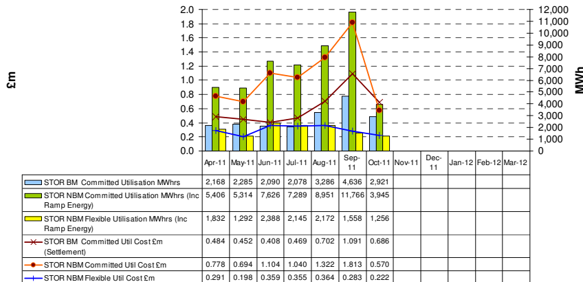
STOR BM & NBM Utilisation MWhr and Cost
